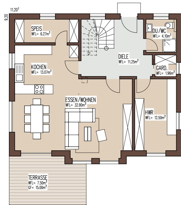
Erdgeschoss
