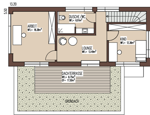
Obergeschoss Variante 1 Einfamilienwohnhaus
