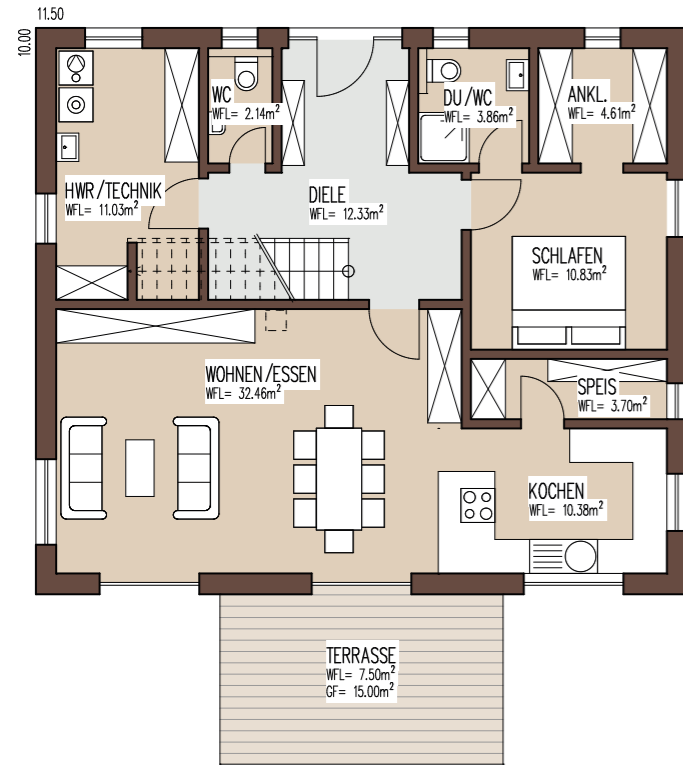
Erdgeschoss
